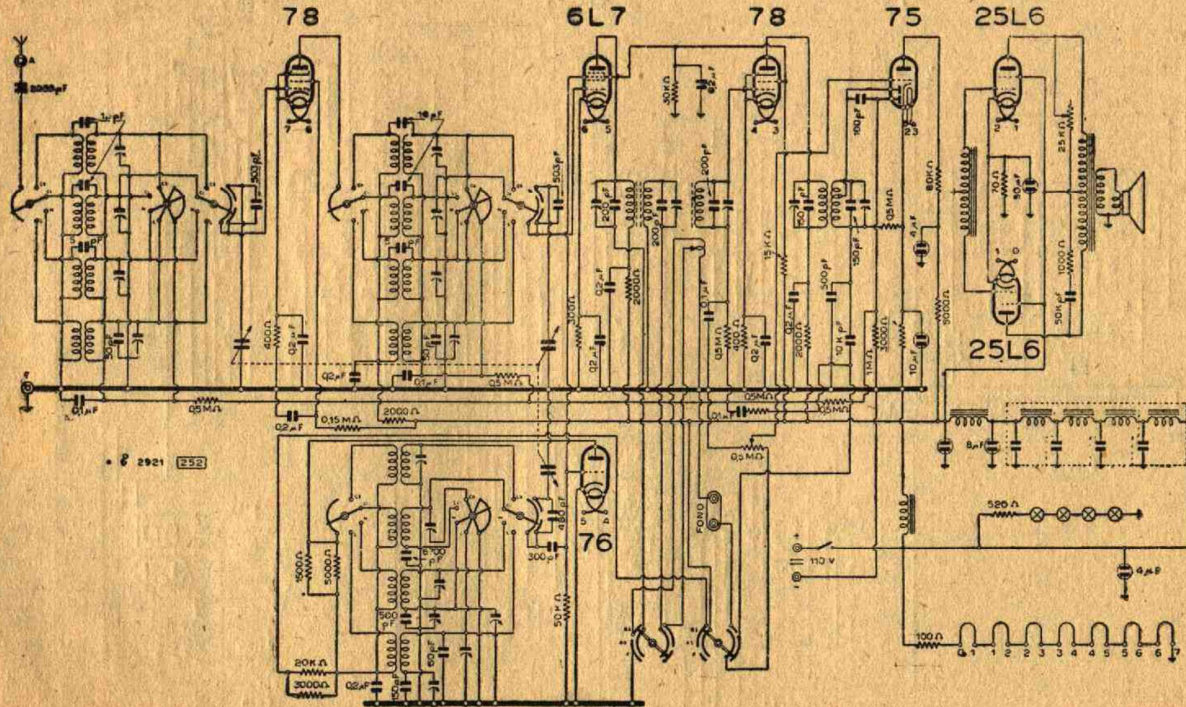
Lo schema elettrico del radiofonografo mod. «748 cc» a corrente continua.
